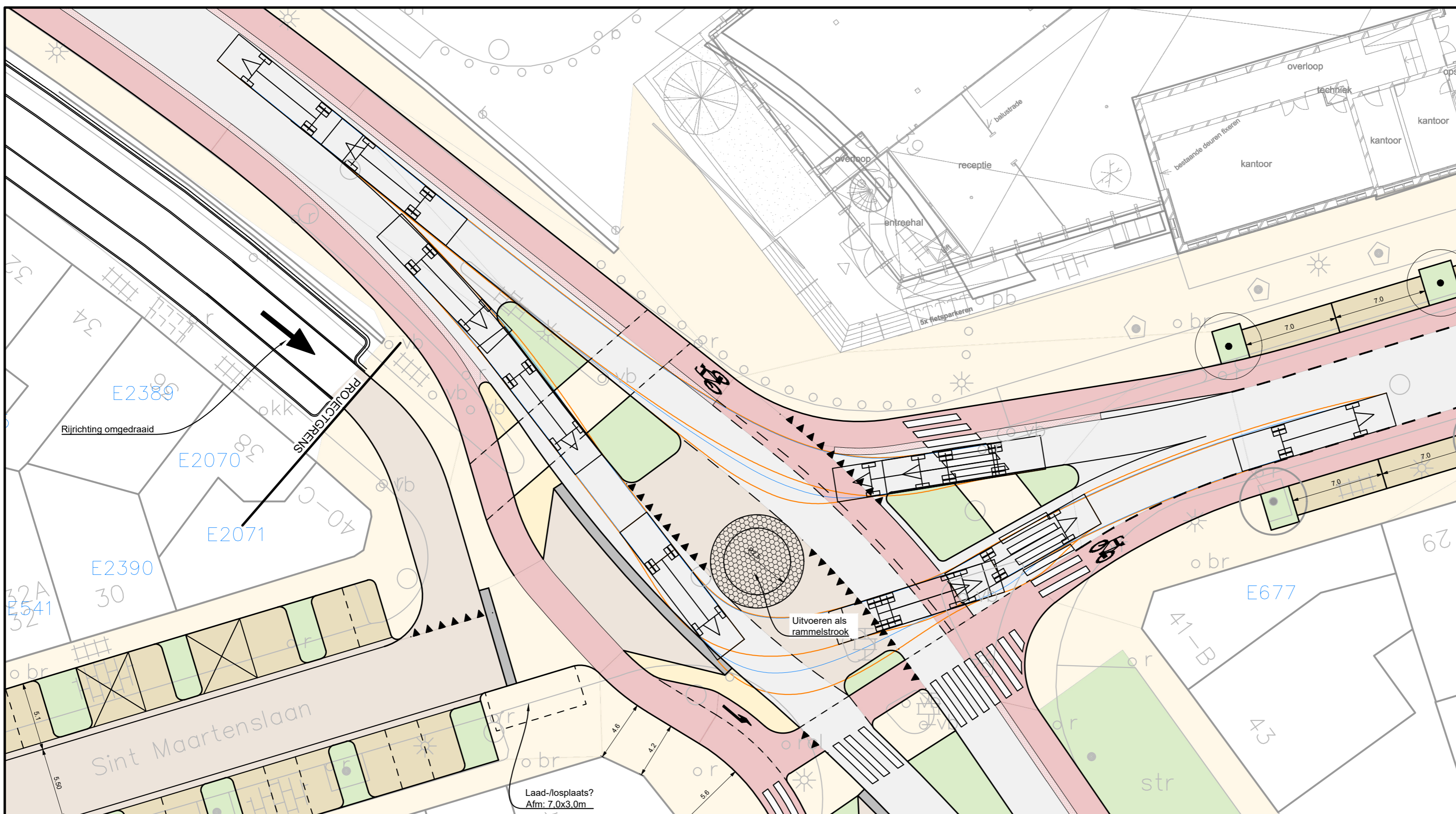
Rijcurvesimulatie bus, lengte 12m
